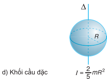
Hình 2.3 Momen quán tính của một số vật đồng chất đối với trục đối xứng \Delta ; m là khối lượng của vật.
