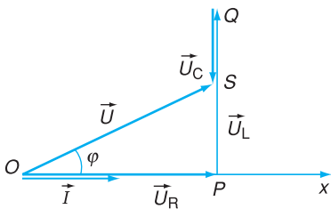
Hình 28.3 Tổng hợp các vector theo quy tắc đa giác.
