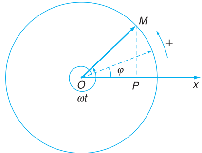
Hình 6.7 Vector quay vào một thời điểm t bất kì.
