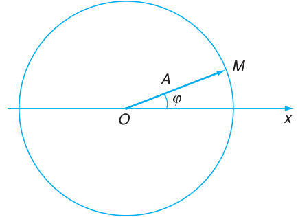
Hình 6.6 Vector quay vào thời điểm t = 0 .
