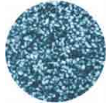
Hình 59.5 Quang cầu.
