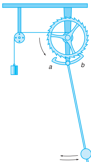
Hình 10.3 Cơ chế duy trì dao động của con lắc.
