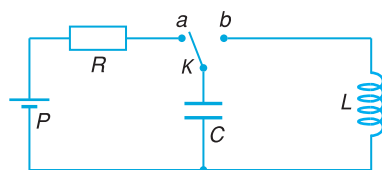
Hình 21.1 Sơ đồ mạch dao động.
