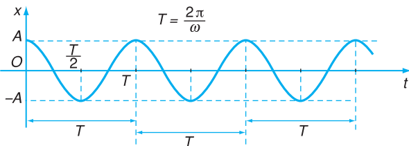
Hình 6.4 Đường biểu diễn x = A\cos(\omega t + \varphi) với \varphi = 0 . Trục hoành biểu diễn thời gian t , trục tung biểu diễn li độ x . A là giá trị cực đại của li độ x .
