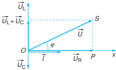
Hình 28.2 Tổng hợp các vector theo quy tắc hình bình hành.
