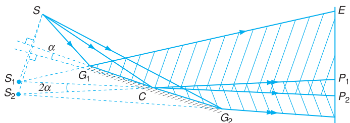
Hình 36.5. Gương Fre-nen.
